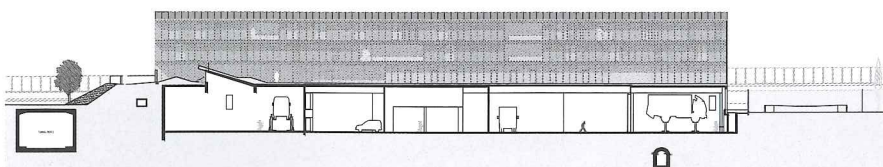
COUPE TRANSVERSALE EST/OUEST ET FAÇADE SUD
