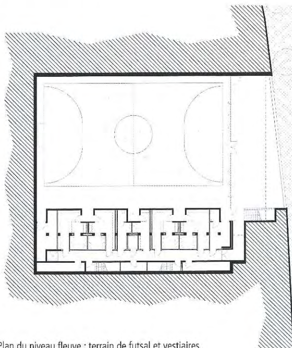
Plan du niveau fleuve : terrain de futsal et vestiaires.
