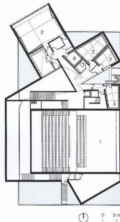
Plan de R+1
